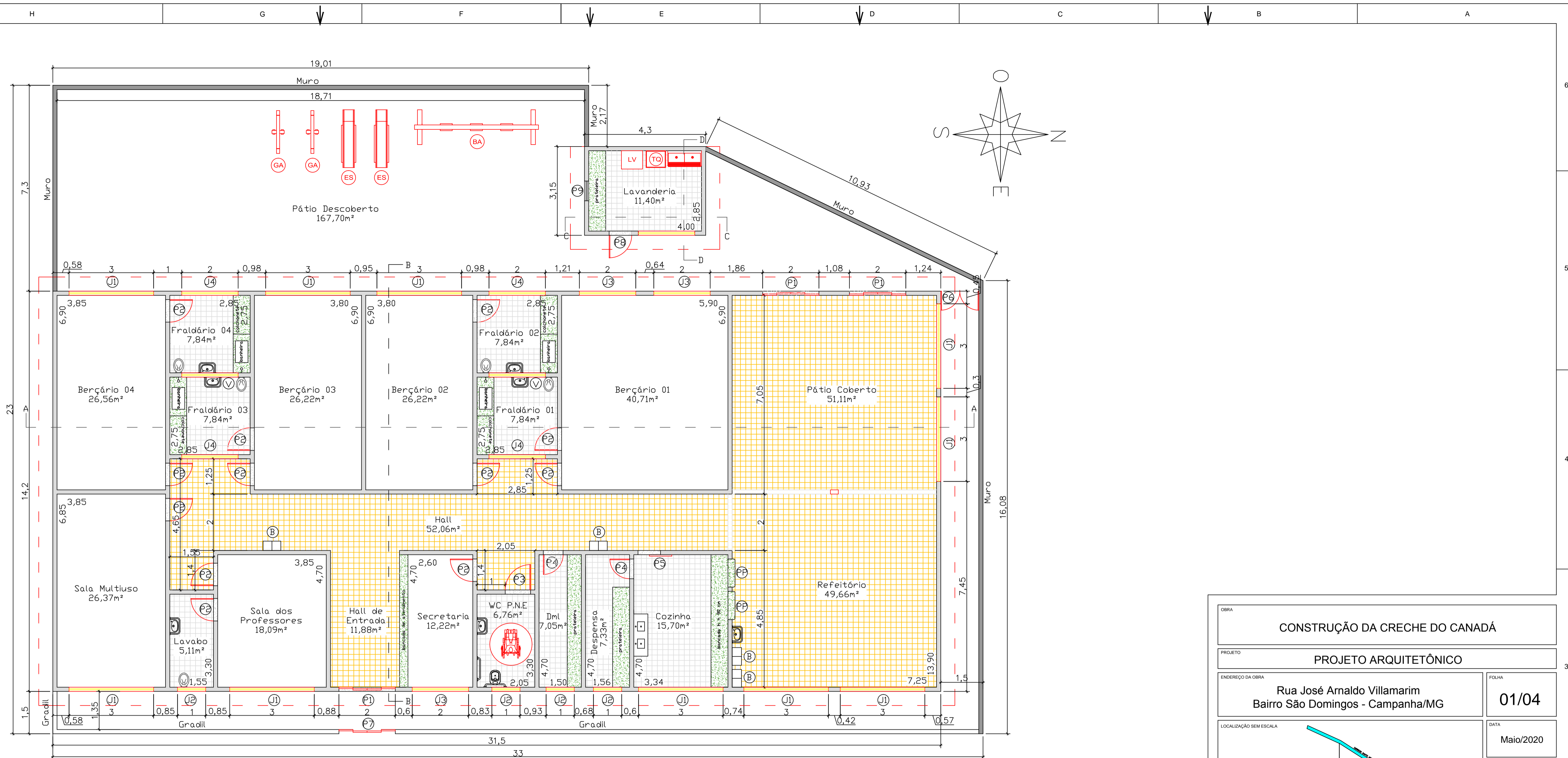
01 PLANTA BAIXA ESCALA 1:75
